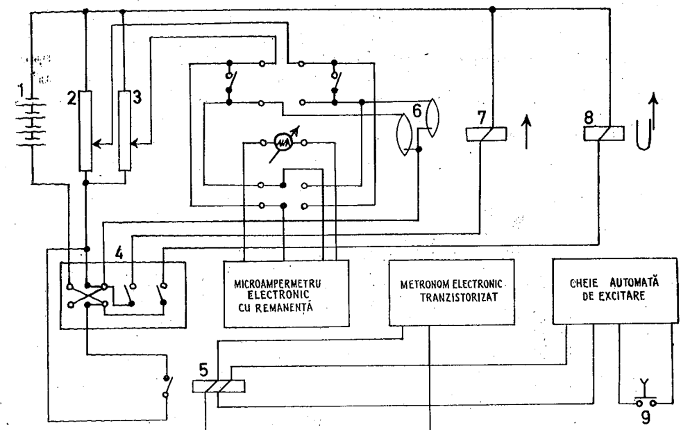
Fig. 1. — Schema generală de principiu a circuitului de excitație. 1, Sursă de curent continuu; 2 și 3, reostate; 4, întrerupătoare pentru circuitul de excitație; 5, relee electro-magnetic; 6, mușchi gastrocnemieni; 7, semnal electric; 8, cronograf diapazon; 9, cheie manuală.
