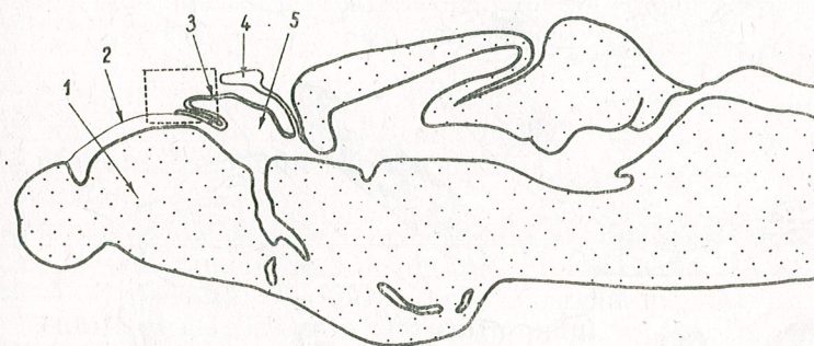
Fig. 1. — Schemă reprezentând o secțiune sagitală prin encefal de Carassius , pentru a pune în evidență locul de unde s-a recoltat materialul: 1, ganglioni bazali; 2, pînza coroidiană; 3, plexul coroid; 4, epifiza; 5, ventriculul al III-lea.
