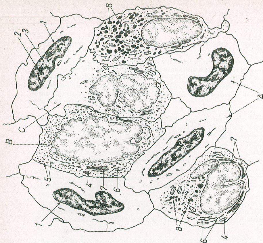
Fig. 3. — Schemă reprezentând tipurile de celule din pinza coroidiană: A, celulă de tip I; B, celulă de tip II; C, celulă de tip III. 1, nucleu cu aspect picnotic; 2, heterocromatină; 3, eucromatină; 4, ergastoplasmă; 5, mitocondrii; 6, corpi multiveziculi; 7, vezicule pinocitare; 8, expansiune voluminoasă de citoplasmă; 9, joncțiuni intercelulare; 10, membrana bazală.
