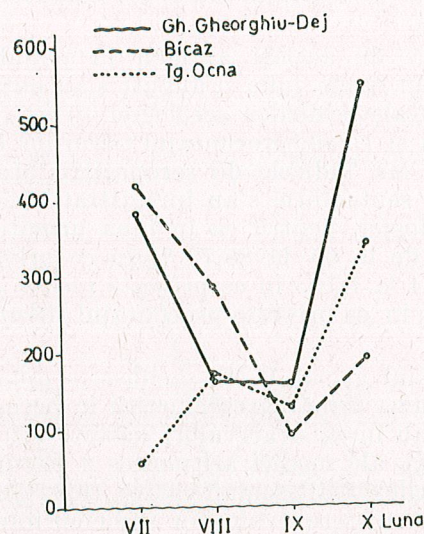
Fig. 6. — Cinetica mediei aritmetice a titrurilor HAI față de antigenul gripal B/Massachusetts 3/66.
