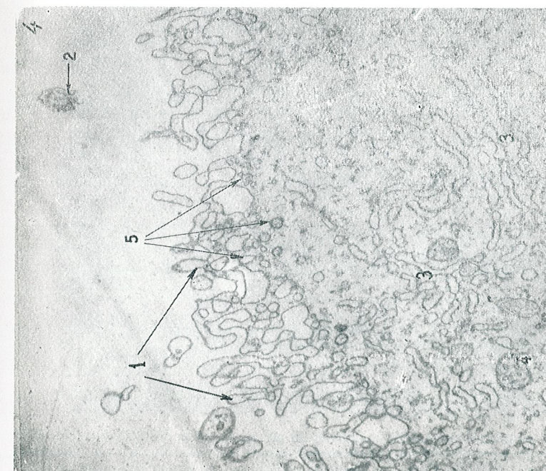
Fig. 4. — Polul apical al unei celule epiteliale din plexul coroid de la Carassius : 1, microvilozități neregulate; 2, cil; 3, ergastoplasmă; 4, corp multivezicular; 5, vezicule de pinocitoză.
