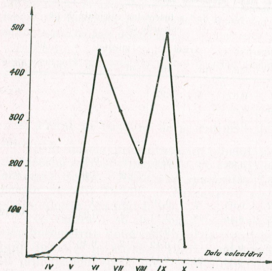
Fig. 1. — Dinamica speciilor de cicadine colectate de pe culturile de lucernă (Cluj, 1956—1970).
