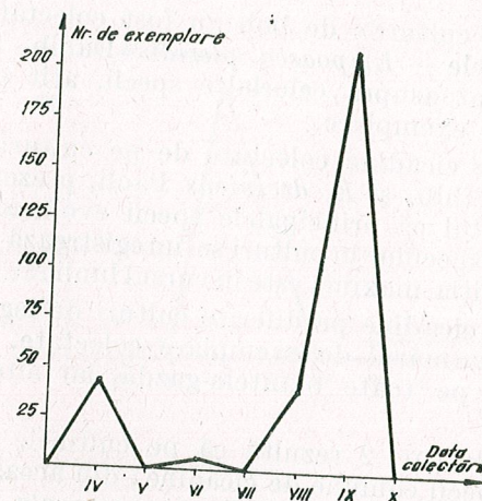
Fig. 5. — Dinamica speciei Macrosteles laevis Rib., pe culturile de trifoi (Cluj, 1956—1967).
