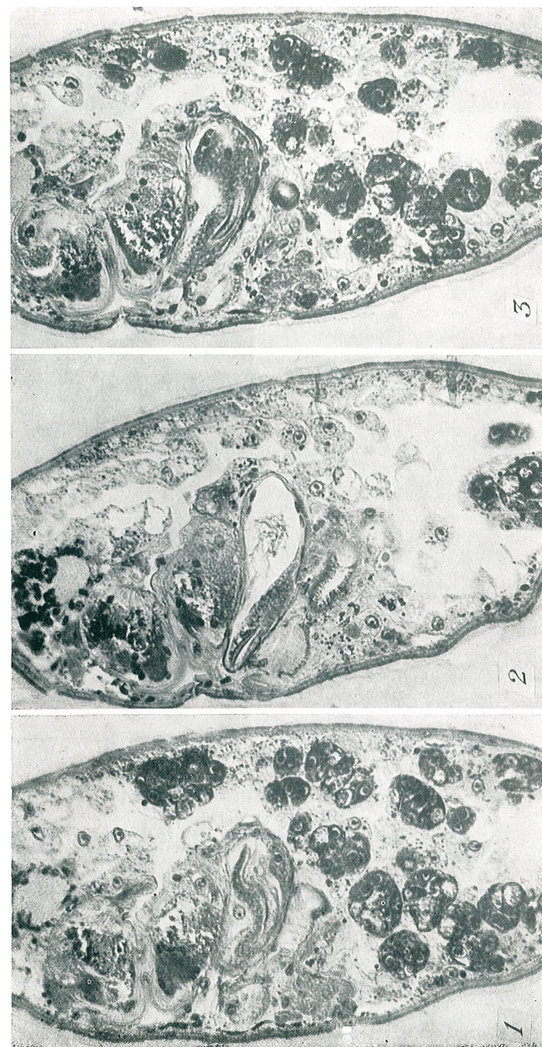
Fig. 1–3. — Strongylostoma sp., trei secțiuni sagitale seriate pentru a se vedea forma ductului ejaculator și separarea atrului genital într-un atrium superius și un atrium inferius (fig. 2).
