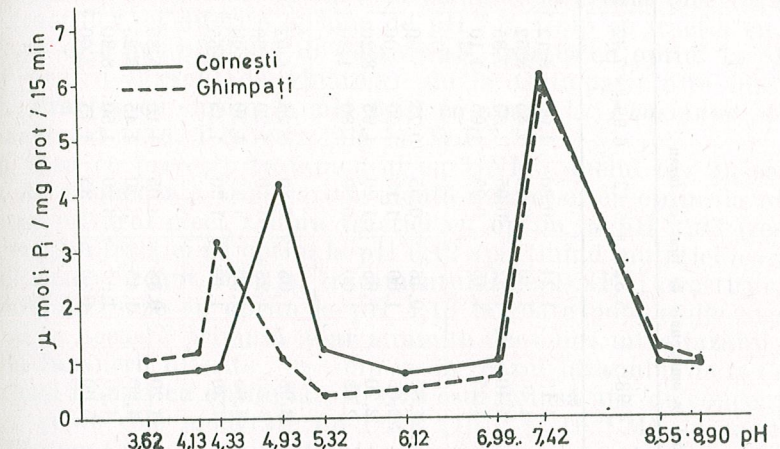
Fig. 1. — Dependența de pH a activității ATP-azice în omogenate de ficat la fazanul de vîntoare ( Phasianus colchicus ) provenit de la fazaneriile Cornești și Ghimpați.
