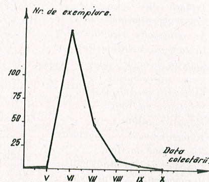
Fig. 2. — Dinamica speciei Aphrodes bi-cinctus Schrk., pe culturile de lucernă (Cluj, 1956—1970).
