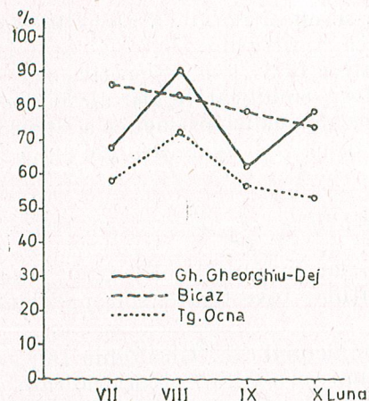
Fig. 7. — Cinetica indicelui de seropozitivitate față de antigenul adenoviral.
