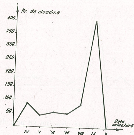
Fig. 4. — Dinamica speciilor de cicadine colectate de pe culturile de trifoi (Cluj, 1960—1967).
