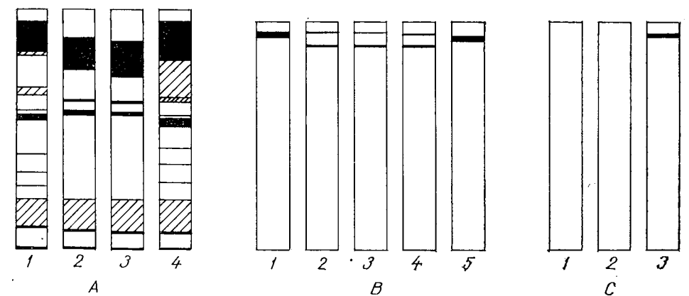
Fig. 4. — Efectul iradierii cu raze X asupra proteinelor serice. A, ser diluat 1:4 (1, martor; 2, animal iradiat cu doza de 100 RX; 3, animal iradiat cu doza de 250 RX; 4, martor); B, proteine hidrosolubile din ficat (1, martor; 2, animal iradiat cu doza de 100 RX; 3, 4, animal iradiat cu doza de 250 RX; 5, martor); C, proteine hidrosolubile din pancreas (1, martor; 2, animal iradiat cu doza de 100 RX; 3, animal iradiat cu doza de 250 RX).
