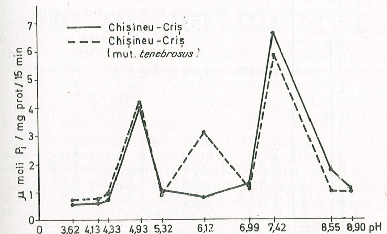
Fig. 2. — Dependența de pH a activității ATP-azice în omogenate de ficat la fazanul de vîntoare ( Phasianus colchicus ) și la mutația tenebrosus ( Phasianus colchicus mut. tenebrosus ), proveniți de la fazaneria Chișineu-Criș.
