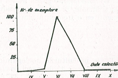
Fig. 10. — Dinamica speciei Empoasca decipiens Paoli, pe culturile de bob (Cluj, 1965—1970).
