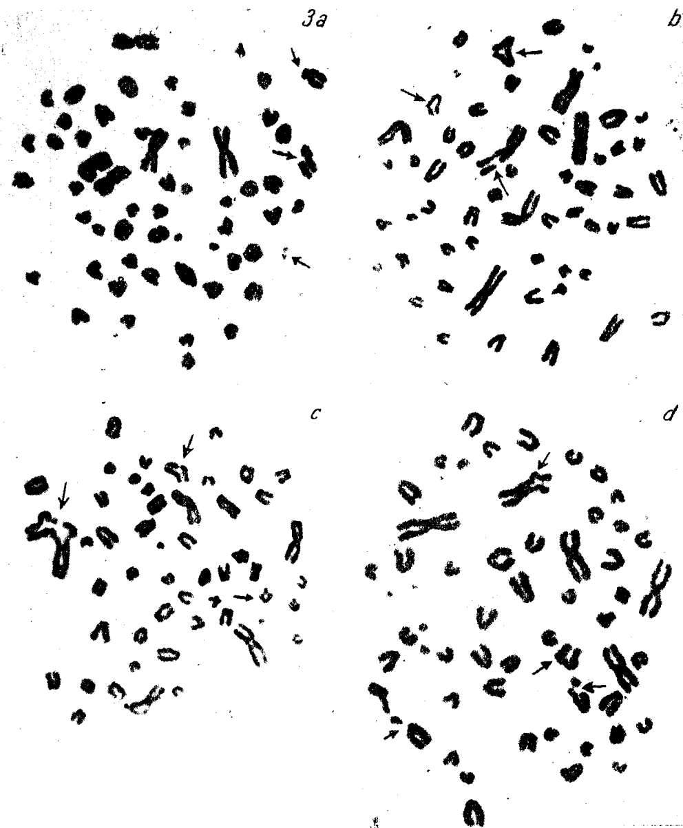
Fig. 3. — Aberrații cromozomiale induse cu doze de 250 RX. a, metafază aneuploidă și translocatii, rupturi cromozomiale și fragmente centrice; b, c, d, metafază cu aberrații multiple (inter- și intraschimburii, ruptură monocromatidică).
