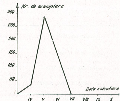
Fig. 8. — Dinamica speciilor de cicadine colectate de pe culturile de bob (Cluj, 1965—1970).
