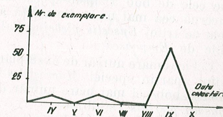
Fig. 6. — Dinamica speciei Tettigella viridis L., pe culturile de trifoi (Cluj, 1956—1967).
