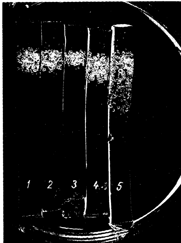
Fig. 5. — Catalaze serice: 1, martor; 2, martor; 3, animal iradiat cu doza de 100 RX; 4, martor; 5, animal iradiat cu doza de 250 RX.
