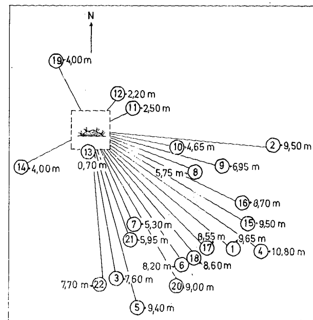
Fig. 1. — Schema biotopului experimental; cifrele încercuite reprezintă denumirea pinilor cercetați, cifrele neîncercuite reprezintă distanțele dintre cuibul de furnici ( Formica pratensis Retz.) și pini.
